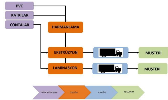
Şekil 1: PVC Profil Üretimi Proses Akış Şeması
